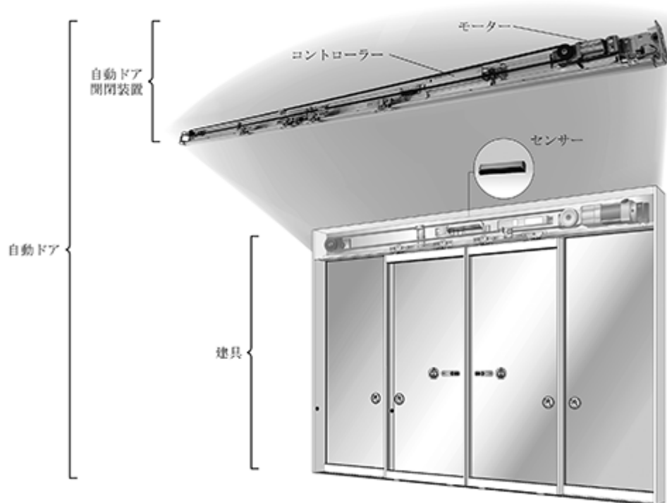
図 - 自動ドア開閉装置と建具の関係図
