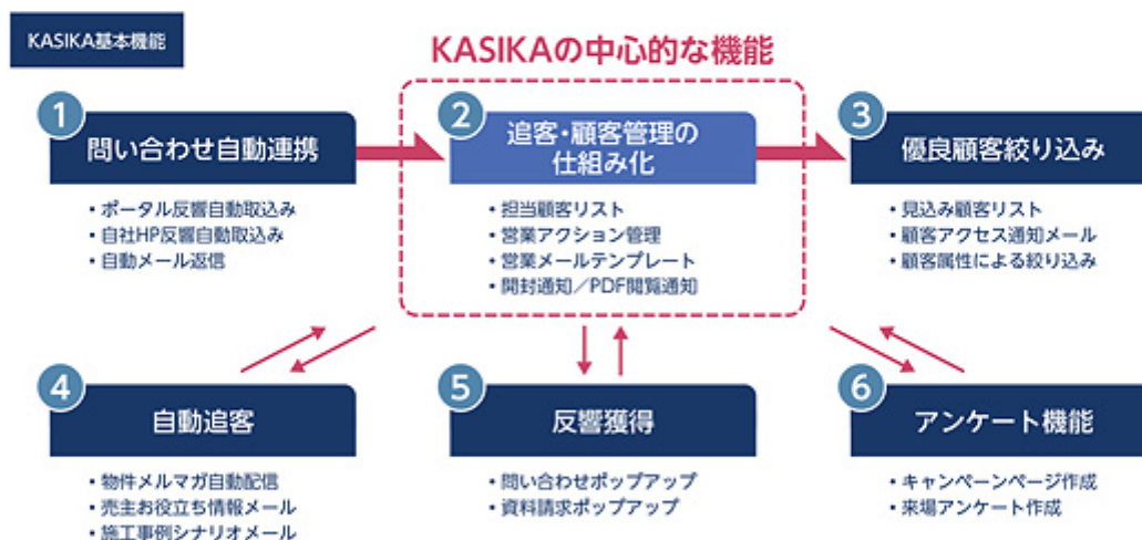
図3: KASIKAの基本機能
