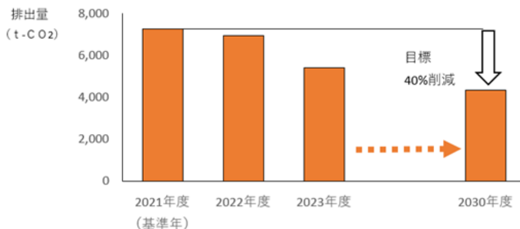
GHG排出量削減イメージ（スコープ1 + スコープ2）
