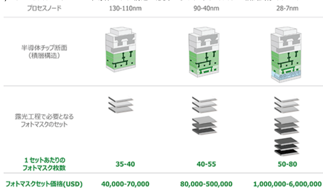
(図4) プロセスノードごとの半導体チップ構造と必要となるフォトマスクの相関関係イメージ
